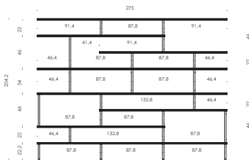
COMPOSITION I L275 D40 H204,2
