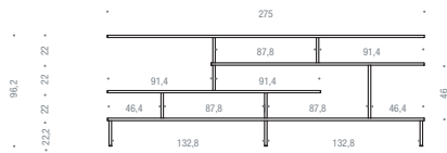
COMPOSITION C L275 D40 H96,2
