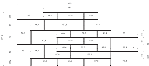
COMPOSITION J L410 D40 H180,2
