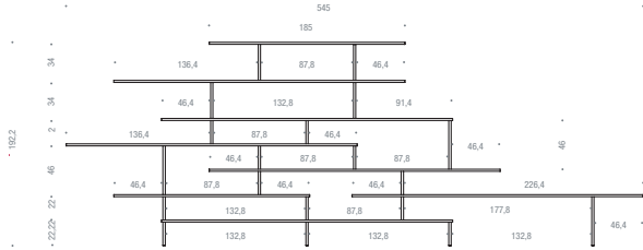
COMPOSITION A L545 D40 H192,2
